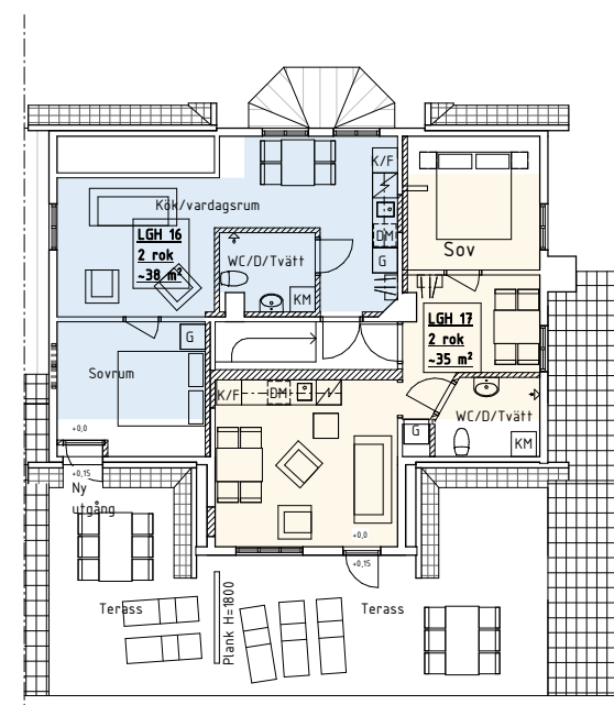
Plan 2 - Ombyggnad
