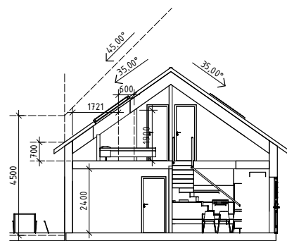
Sektion B
